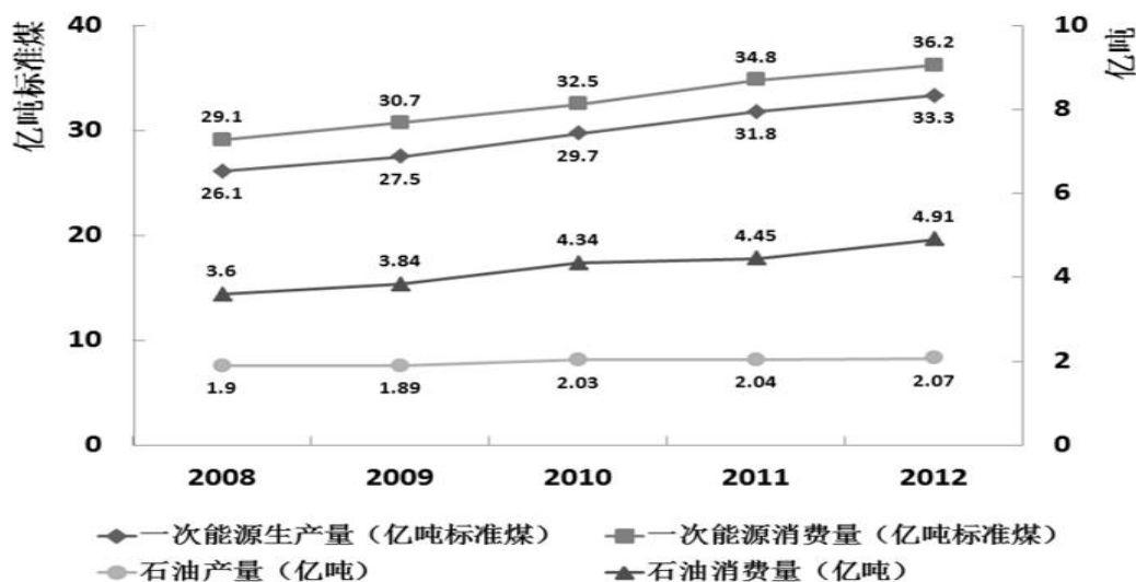
图 1: 2008~2012 年全国一次能源、石油生产量与消费量的情况
